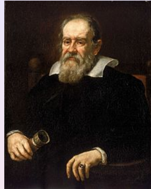
Galileo
