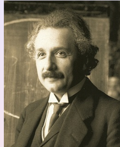
Einstein
