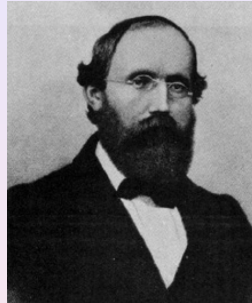
Riemann
